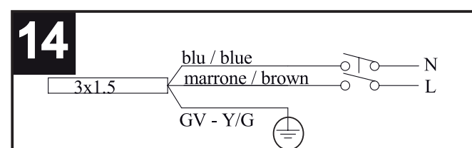
Alimentare (fig.14)
