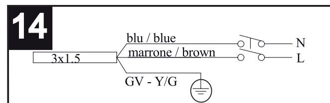
Питание (рис.14)
